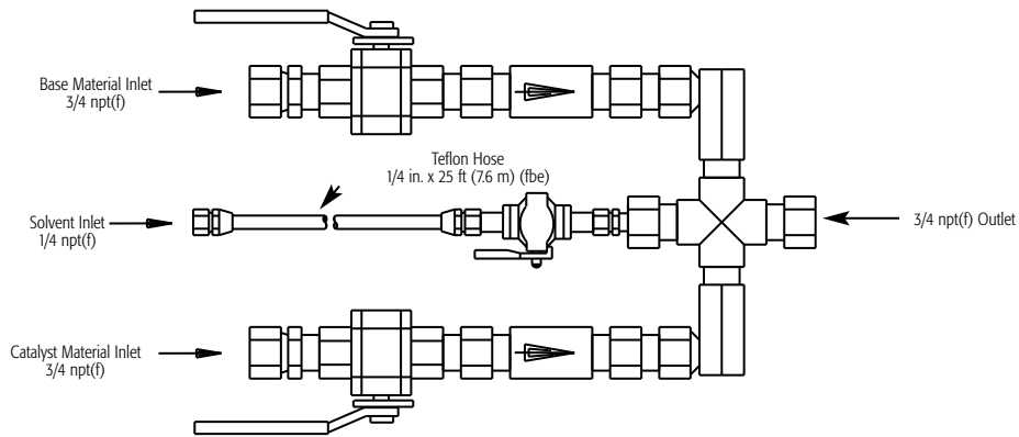
8) High Vol. Static Mix Manifold (570391)
